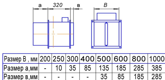
Рис.3. Размеры вылета заслонки в открытом положении за пределы клапана исполнений НЗ-АхВ
