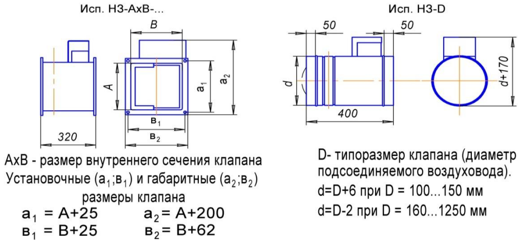
Рис.1. Установочные, габаритные и размеры внутреннего сечения клапана.
